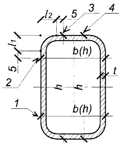
Рисунок 3 – Схема измерения размеров квадратных и прямоугольных профилей
